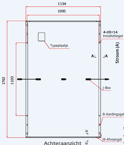
Achteraanzicht
